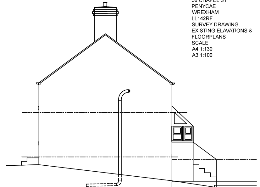
ELEVATION
