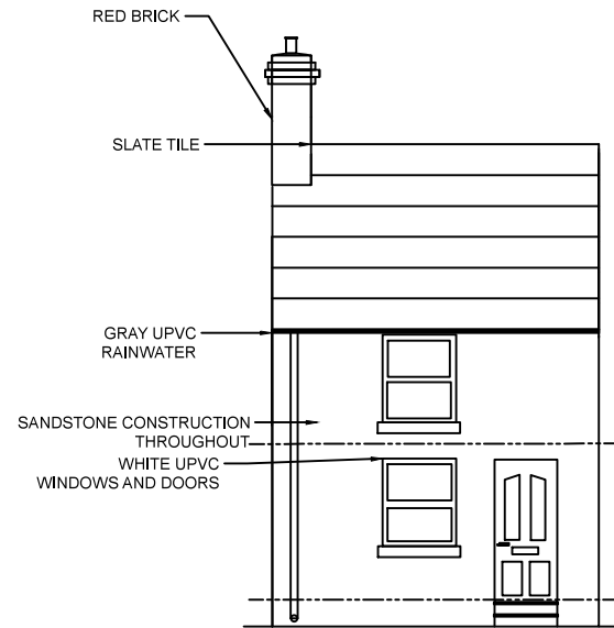
ELEVATION 1
