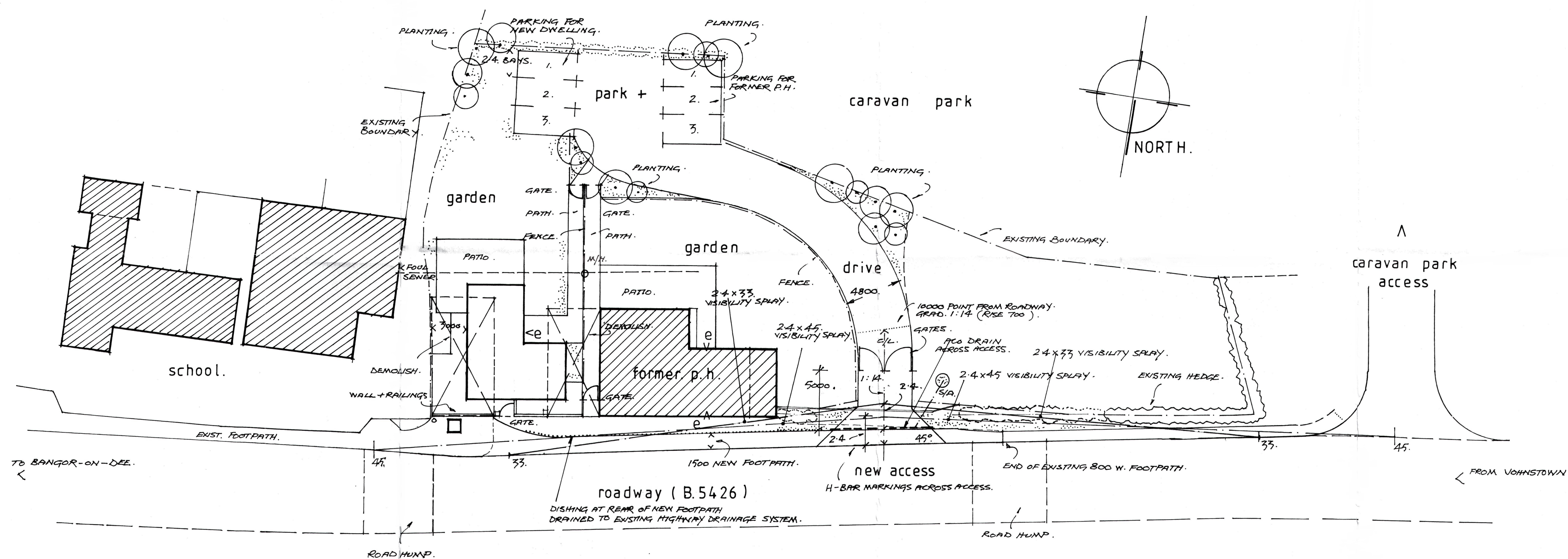
SITE PLAN — 1:200
