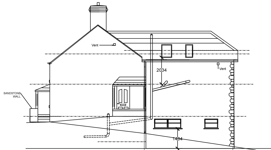
ELEVATION 4
