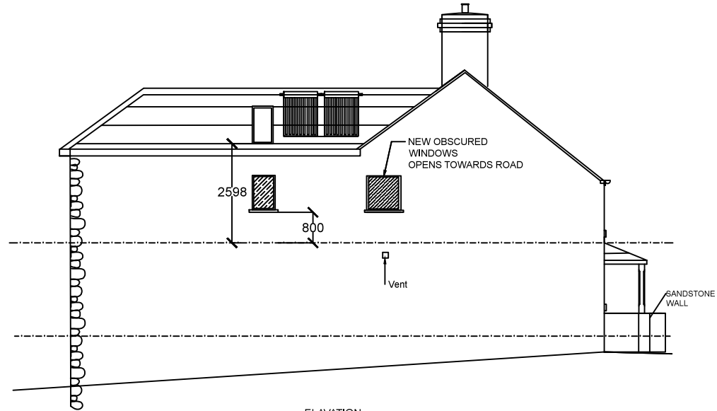
ELEVATION 2
