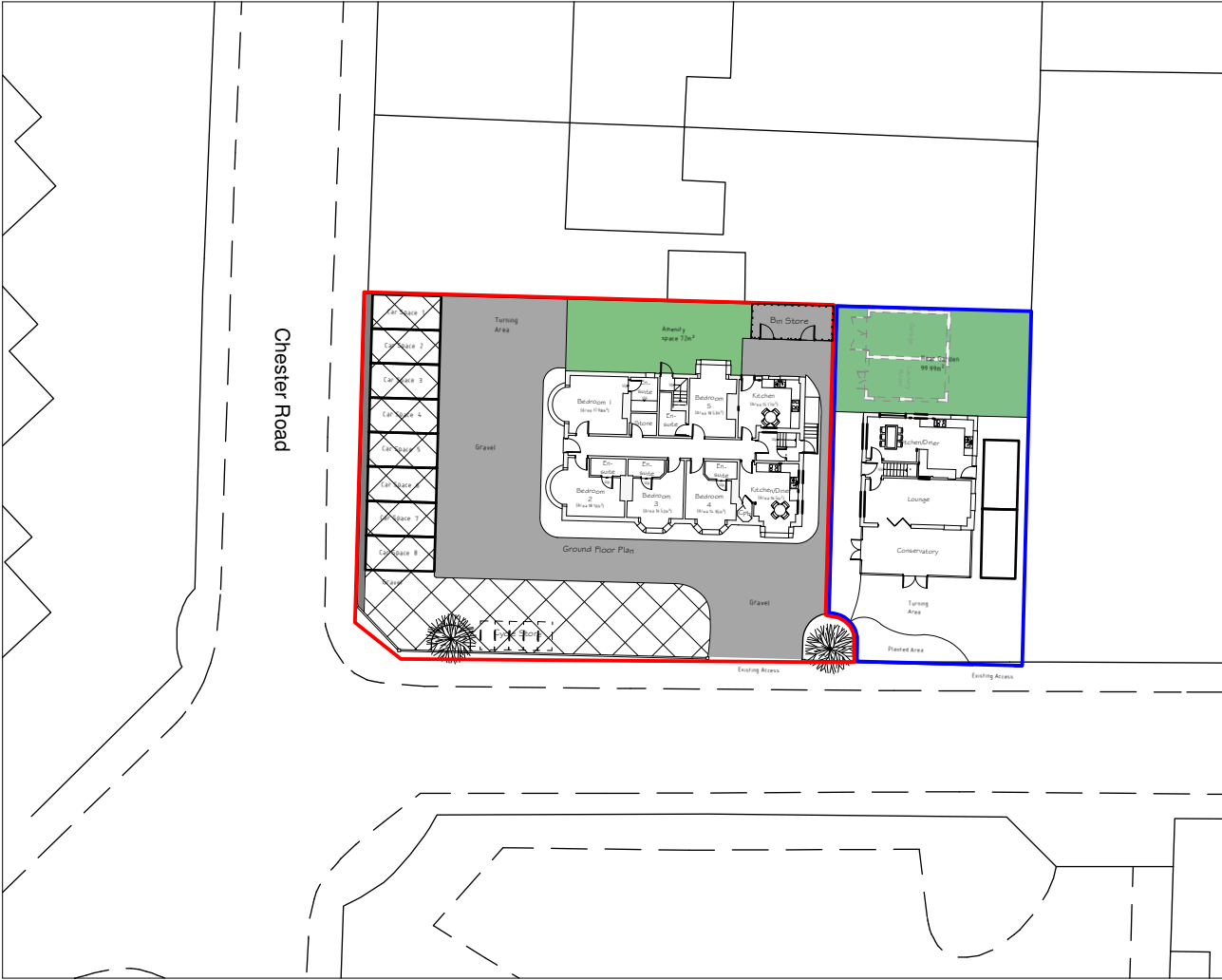
Site Plan 1:500
