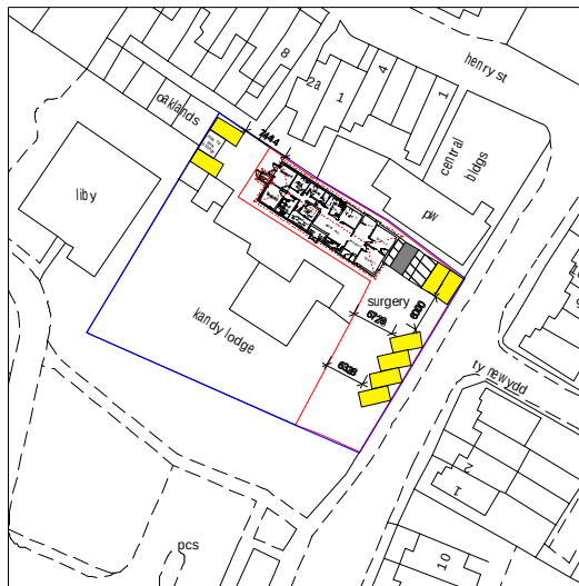
Site Plan 1:500
