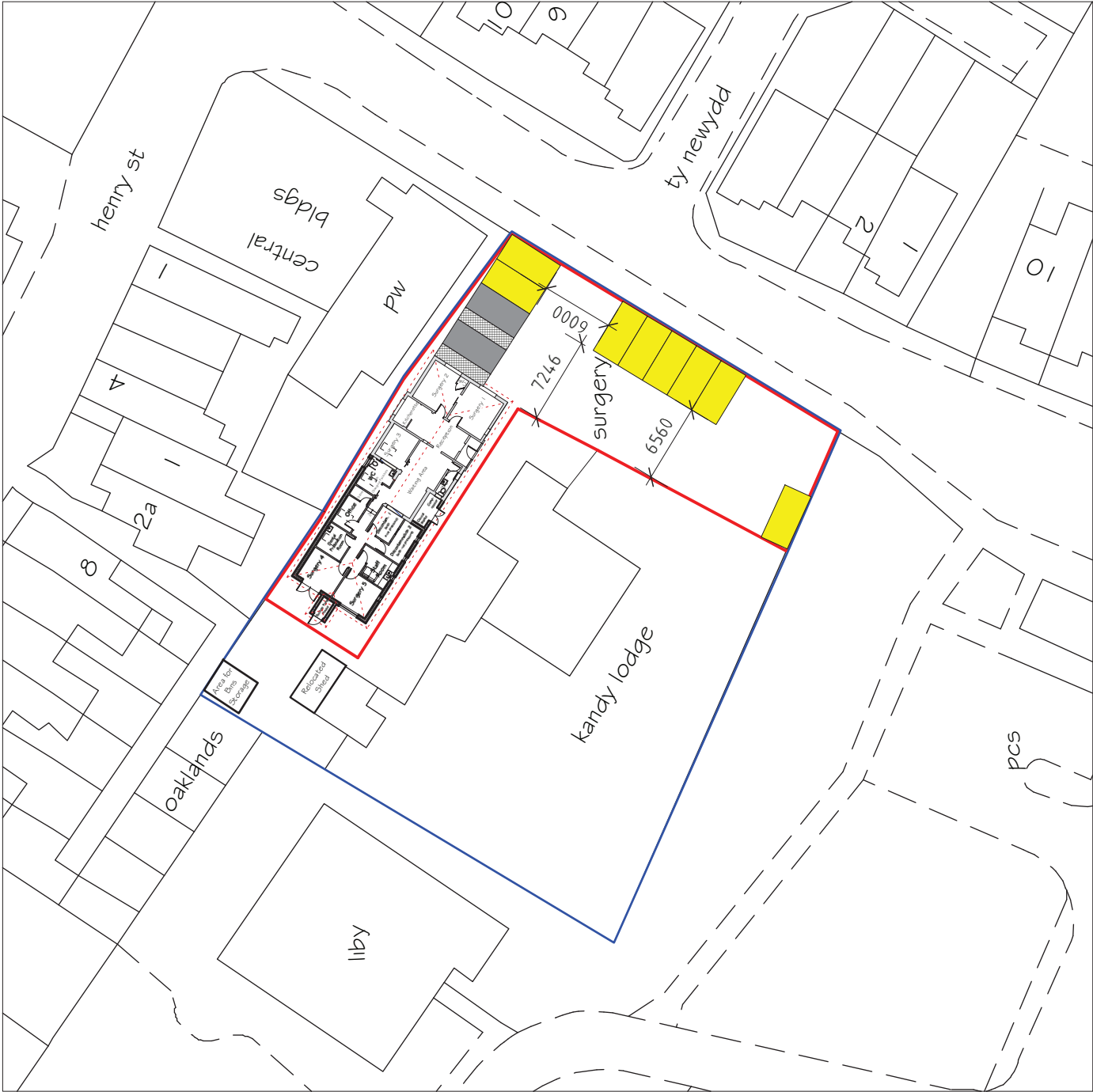
Site Plan 1:500
