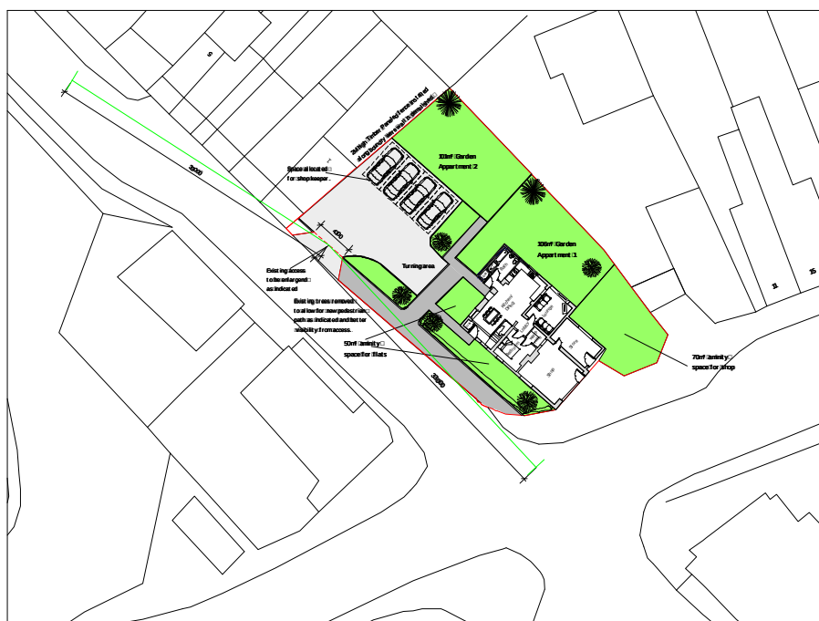
Site Plan 1:200
