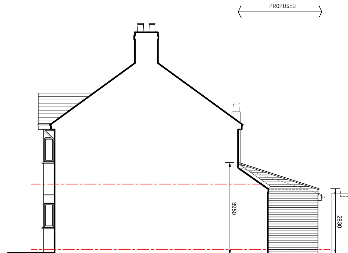
Side-02 elevation 1:100
