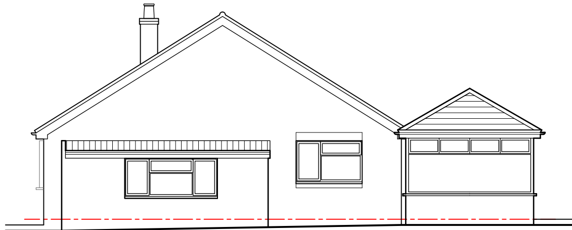
Side-02 Elevation 1:100
