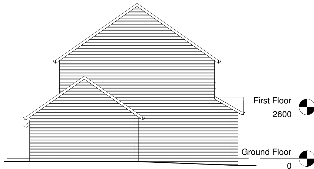
East 1 : 100
