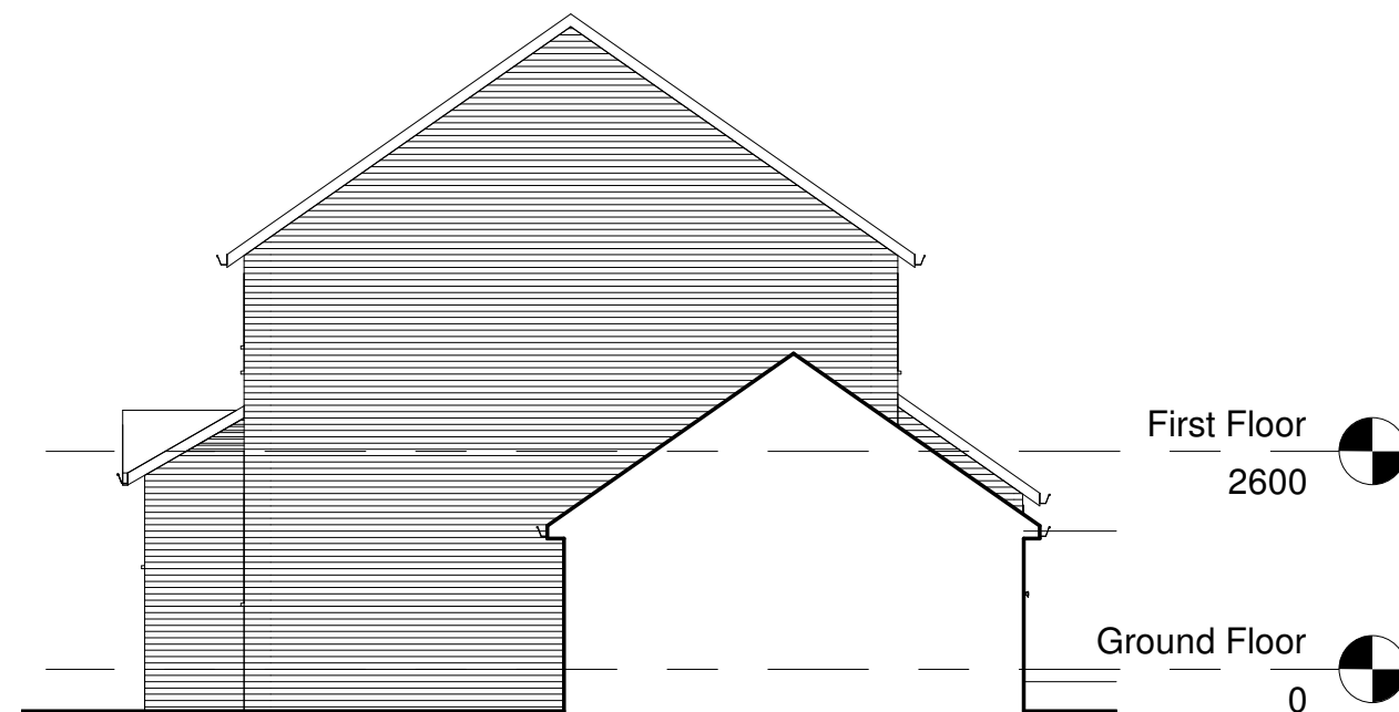
West 1 : 100
