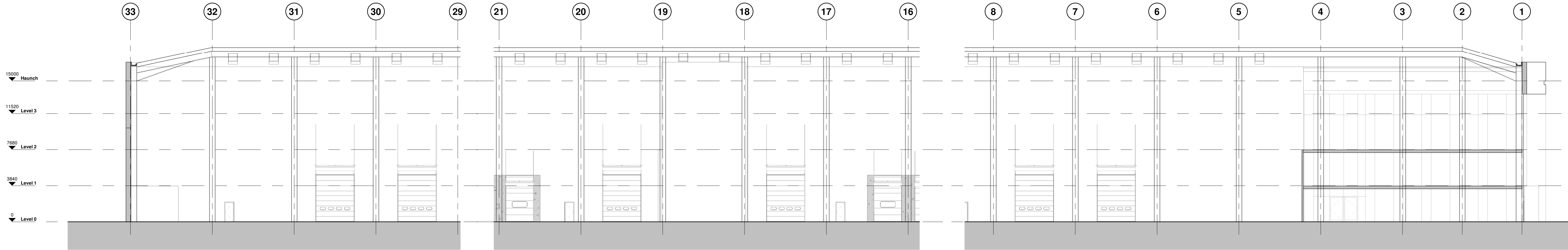
GA-B GA Section B 1 : 200
