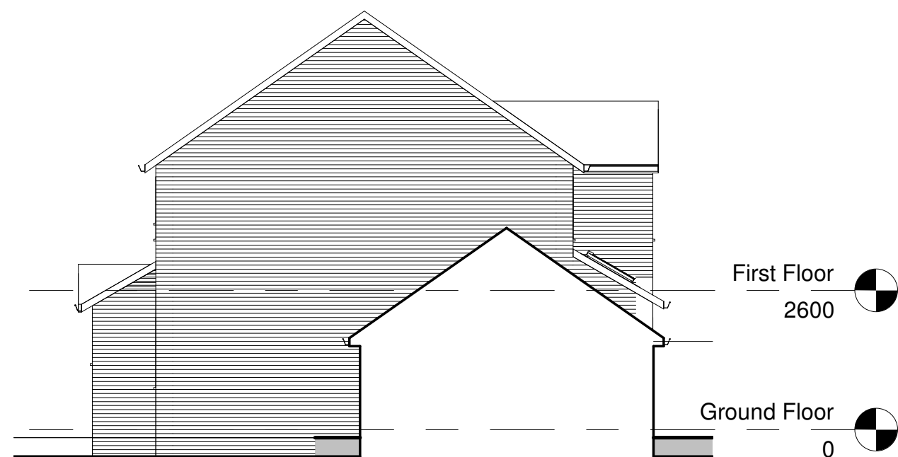
West 1 : 100
