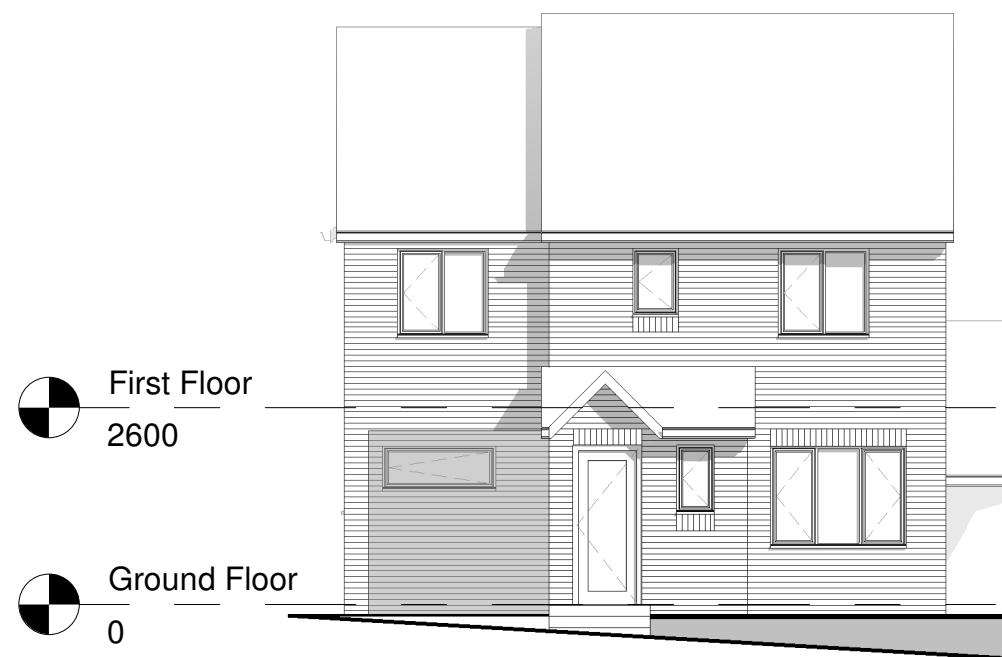
North 1 : 100
