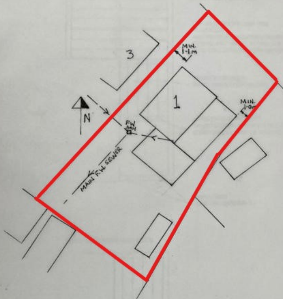
SITE PLAN \approx 1:200
