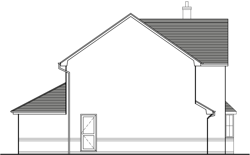
ELEVATION 2
