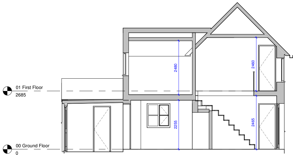
Section 1 1 : 50
