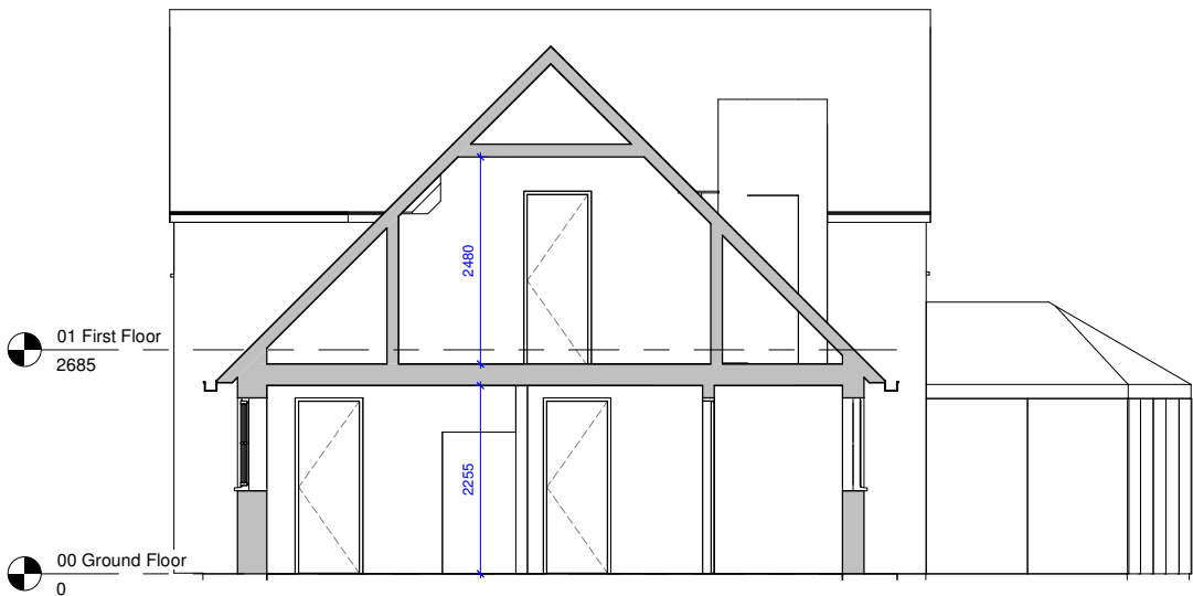
Section 2 1 : 50
