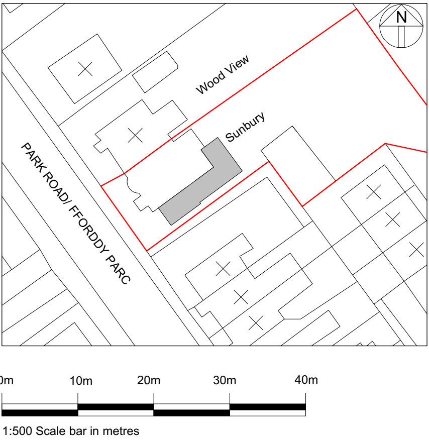
Site Plan 1:500
