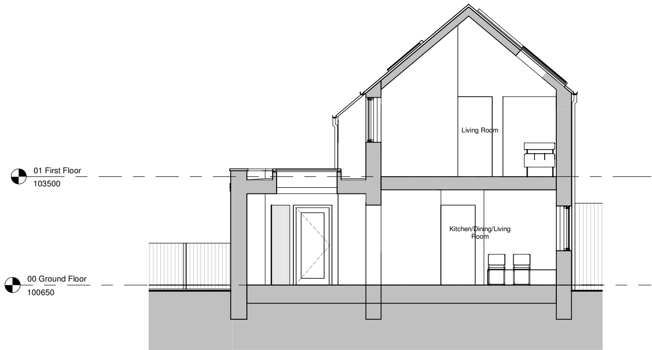
Section B-B 1 : 50 (1 : 100 @ A3)
