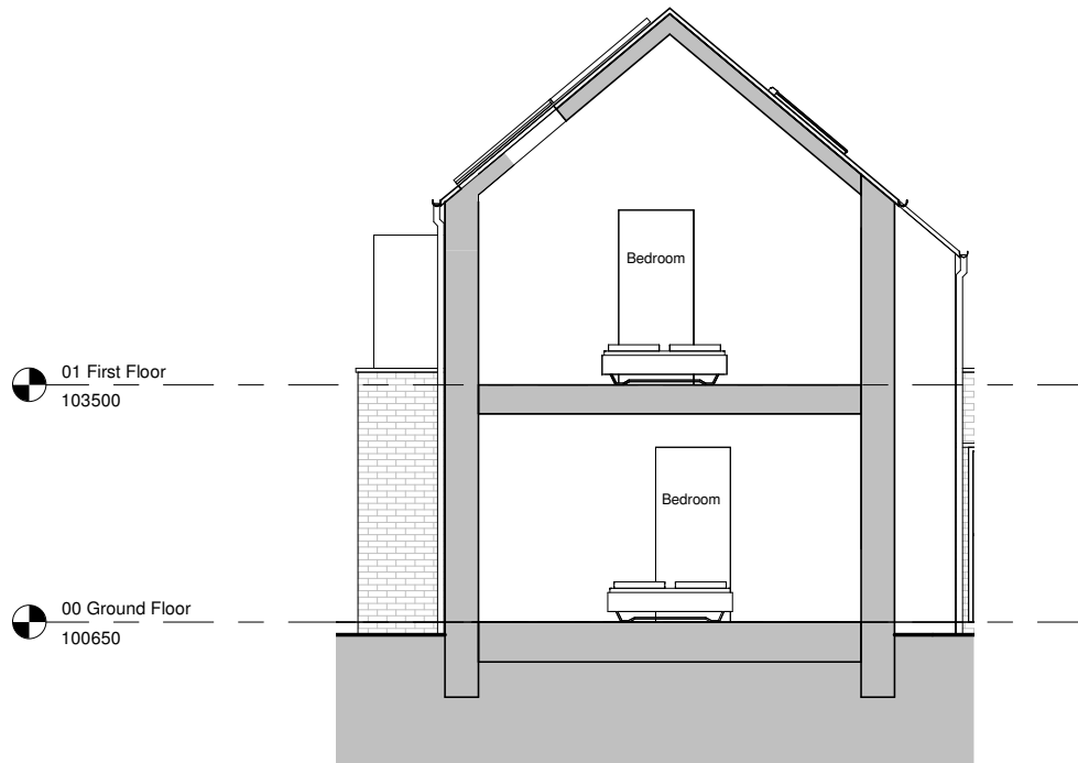
Section C-C 1 : 50 (1 : 100 @ A3)
