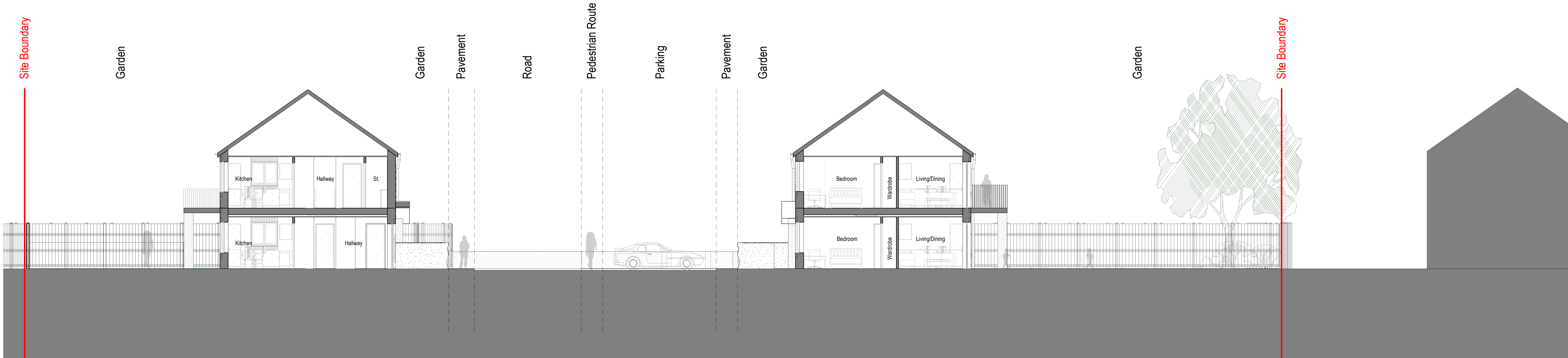
Section 1 1 : 100
