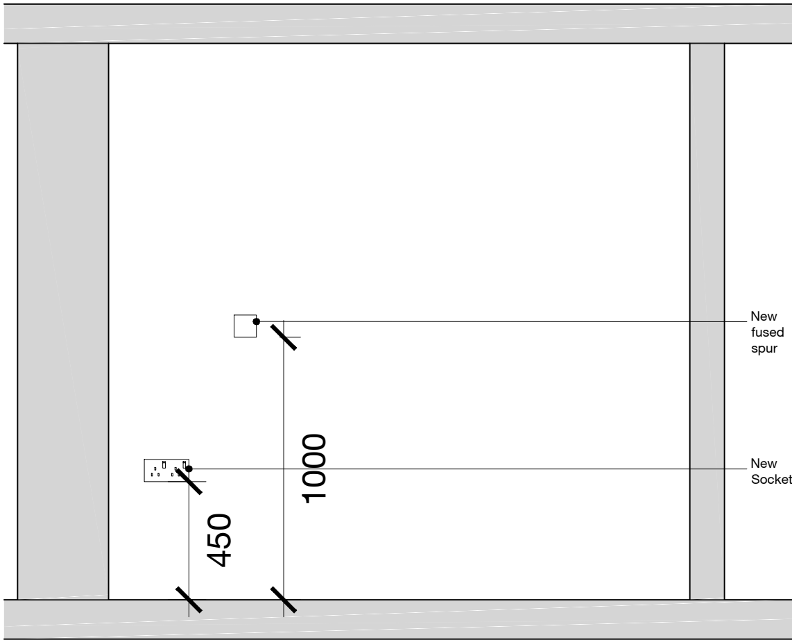
ELEVATION 02
