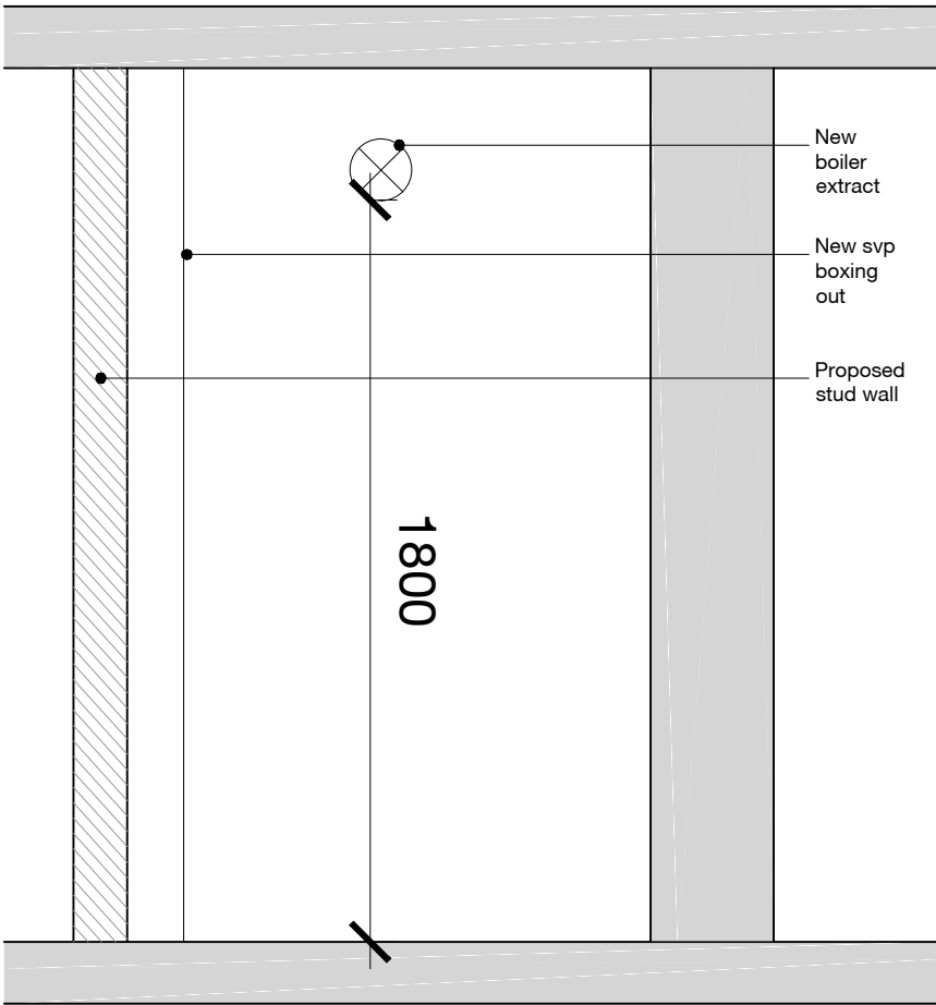
ELEVATION 01
