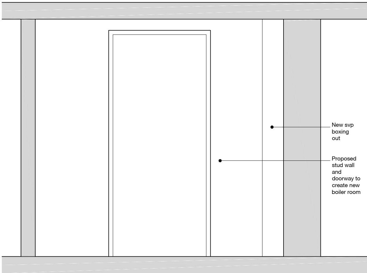
ELEVATION 04
