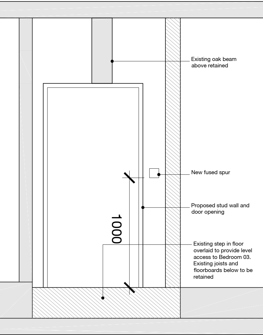
ELEVATION 04
