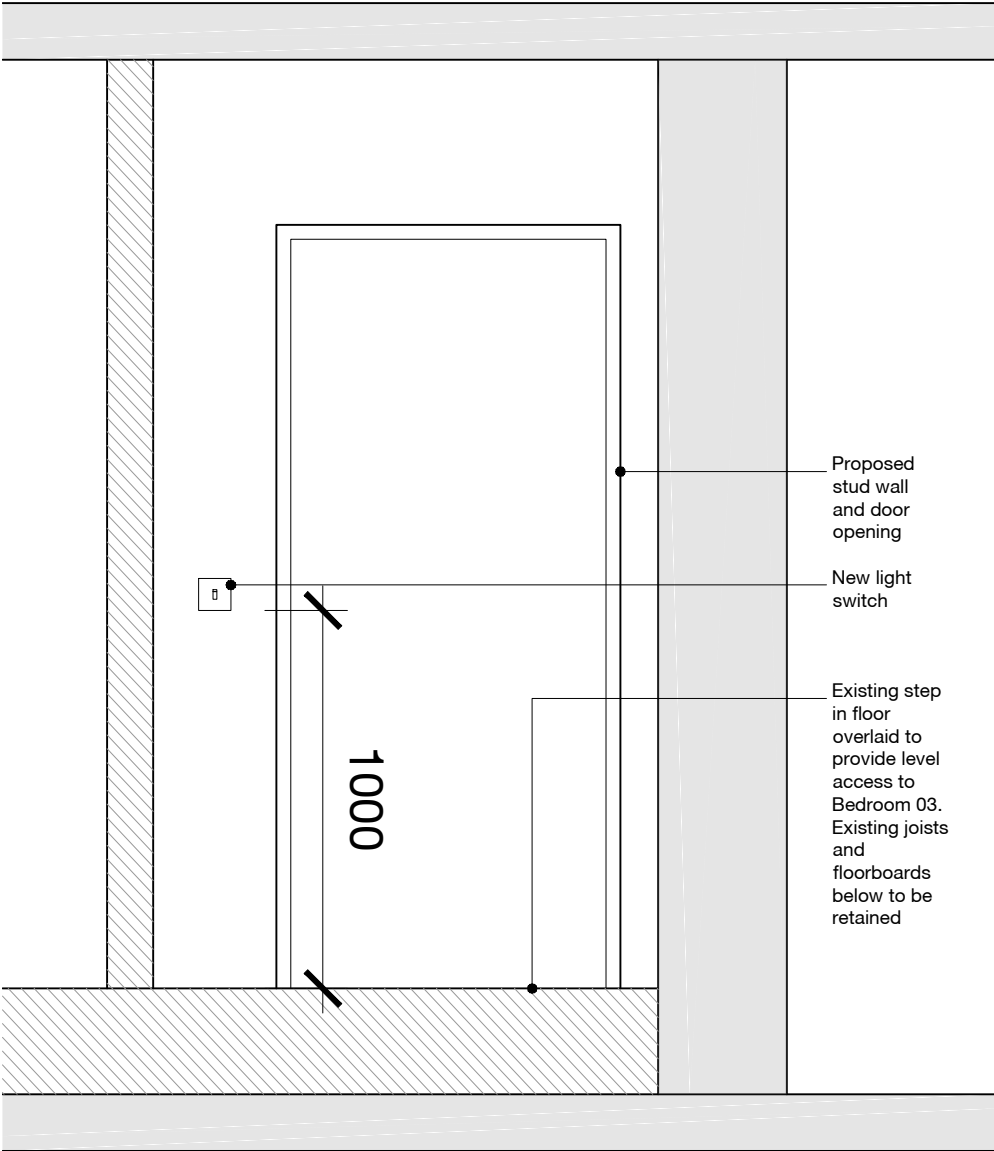
ELEVATION 01
