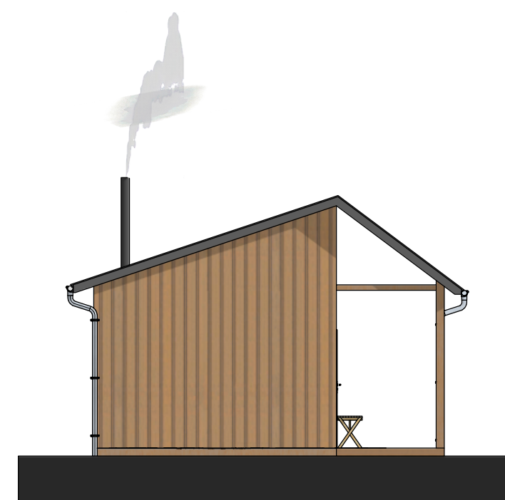
LHS ELEVATION 1:100 @ A1
