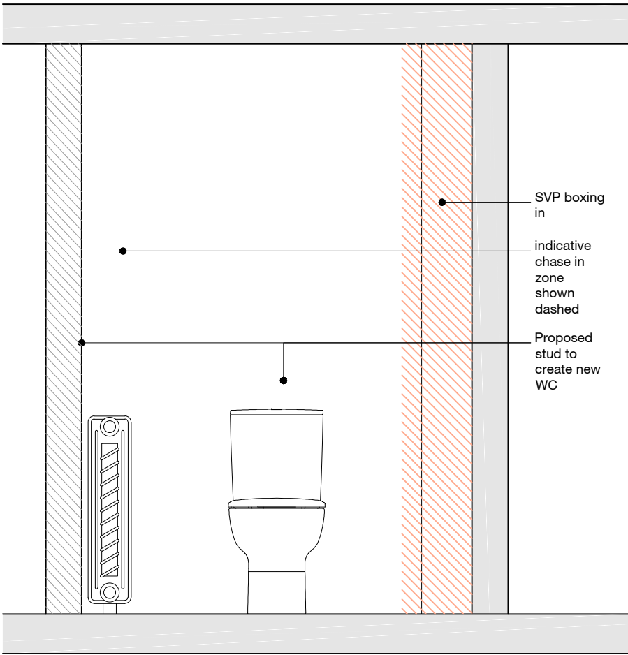
ELEVATION 01
