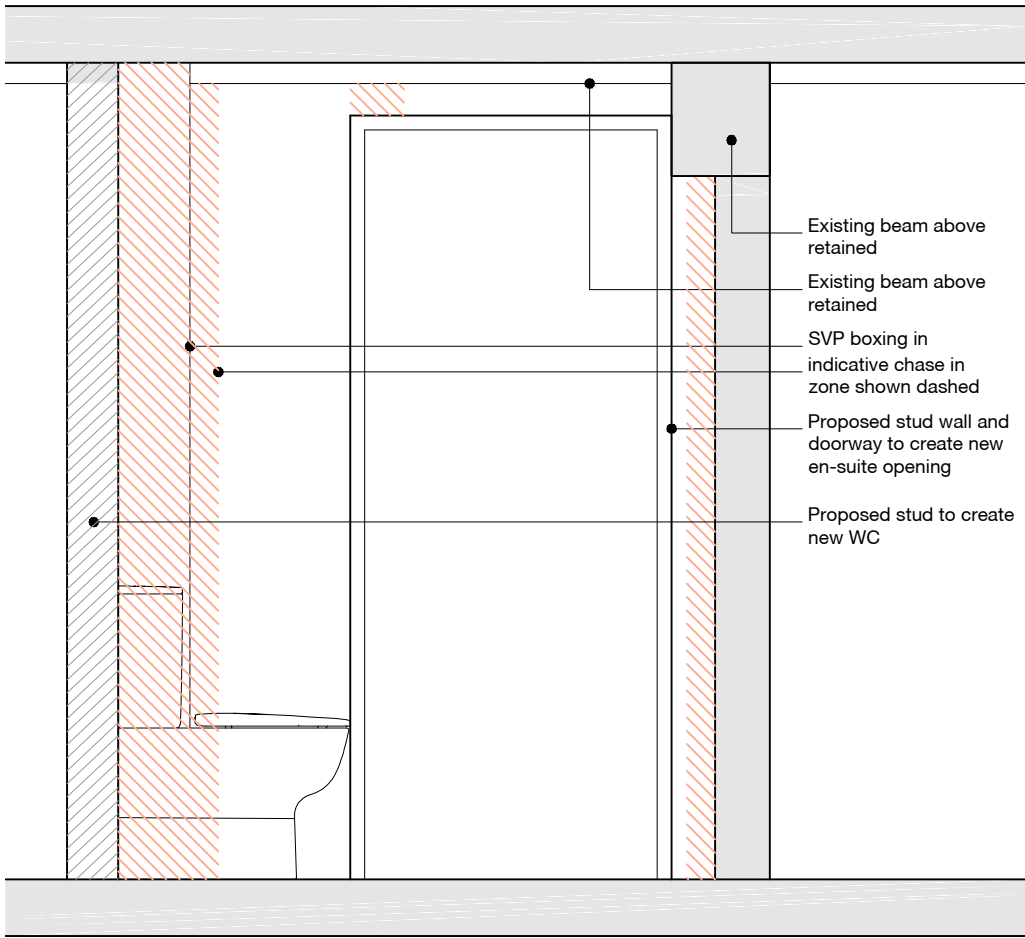
ELEVATION 02
