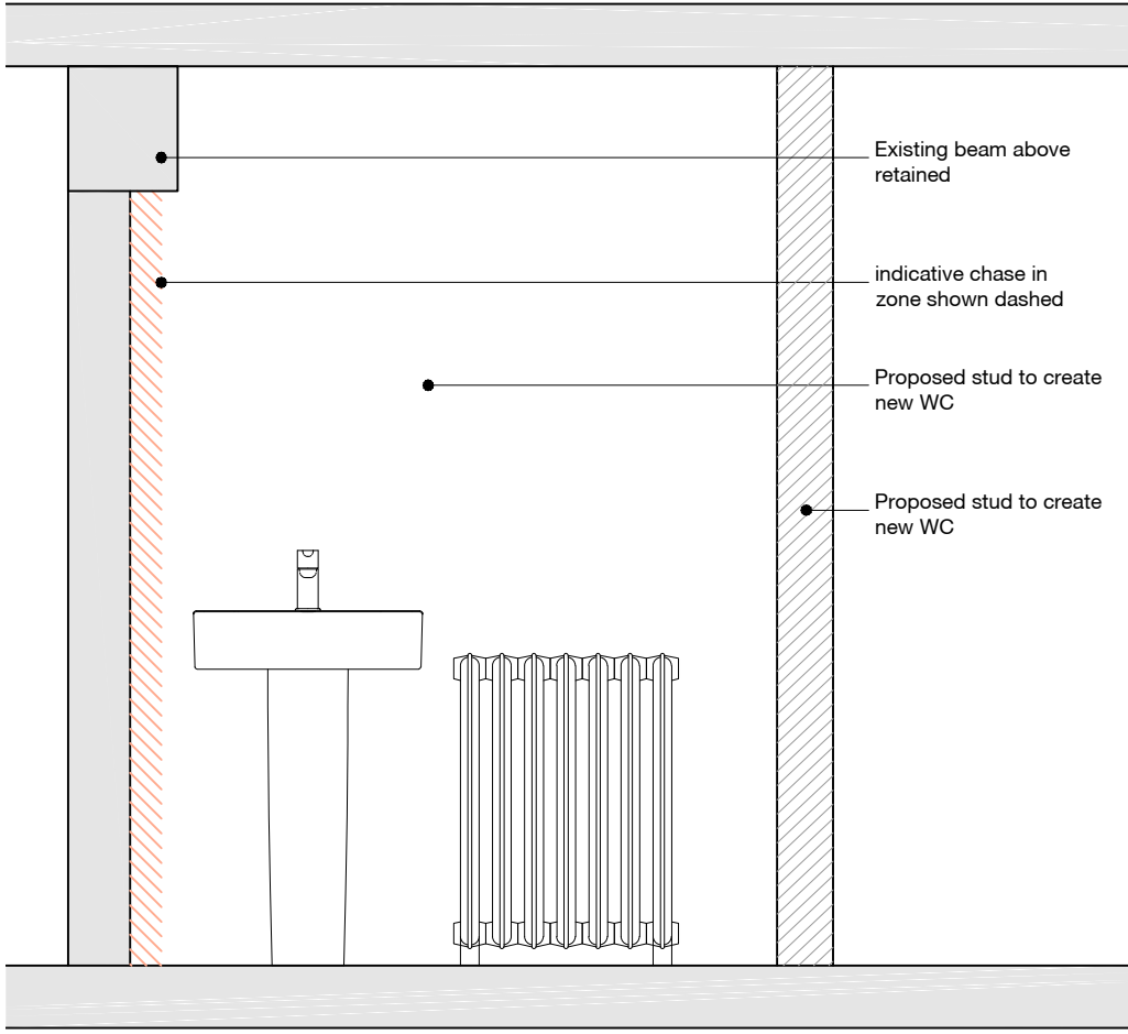
ELEVATION 04
