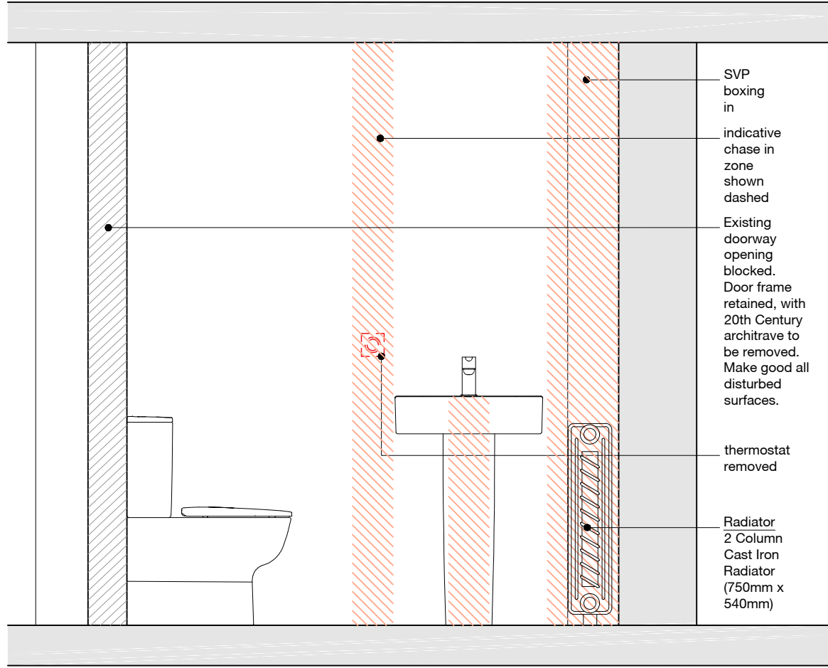
ELEVATION 02
