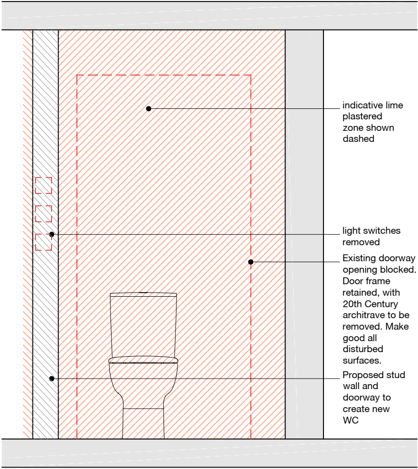
ELEVATION 01
