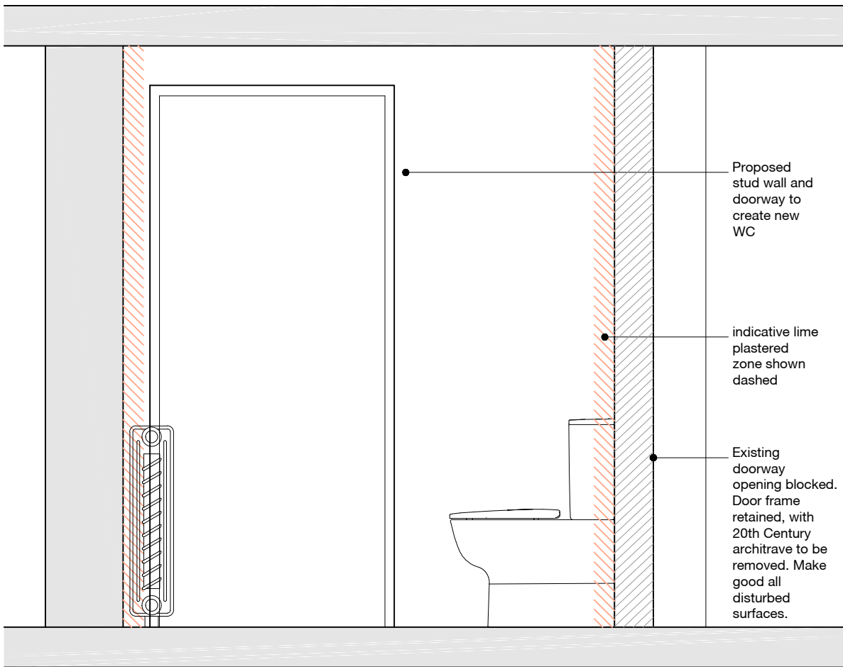
ELEVATION 04
