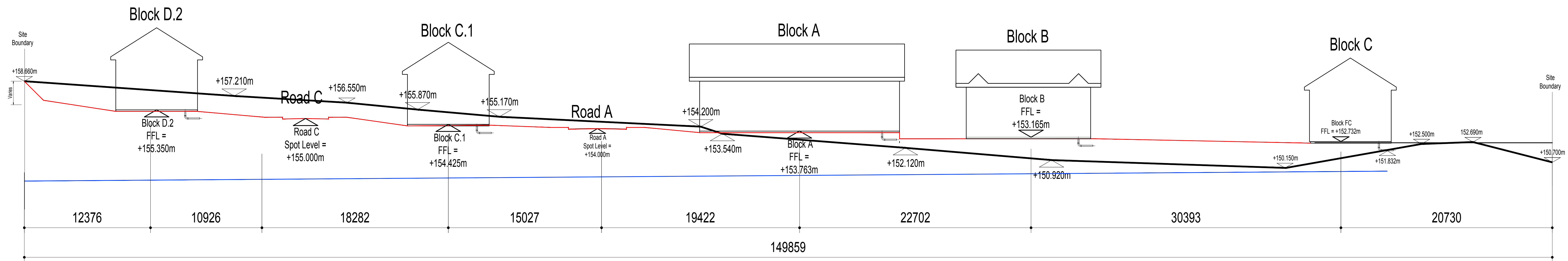
Longitudinal Site Section A-A (1:150)
