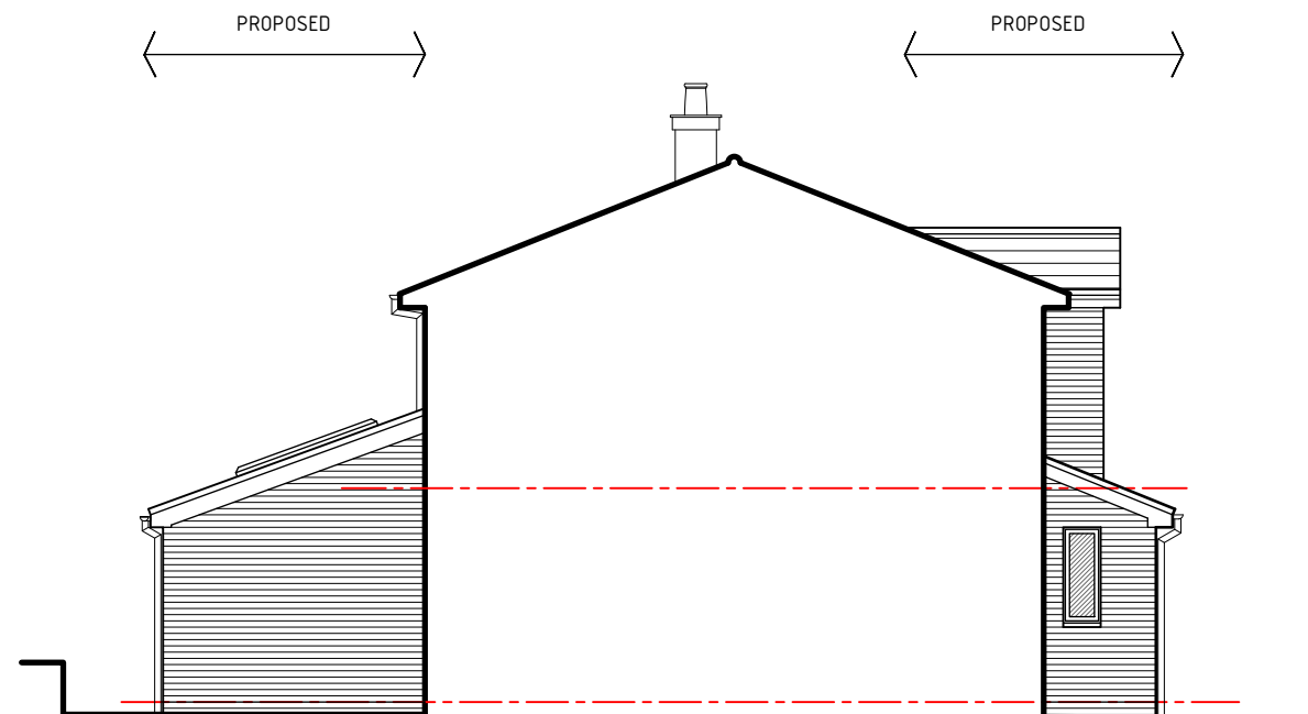
Side-02 Elevation 1:100
