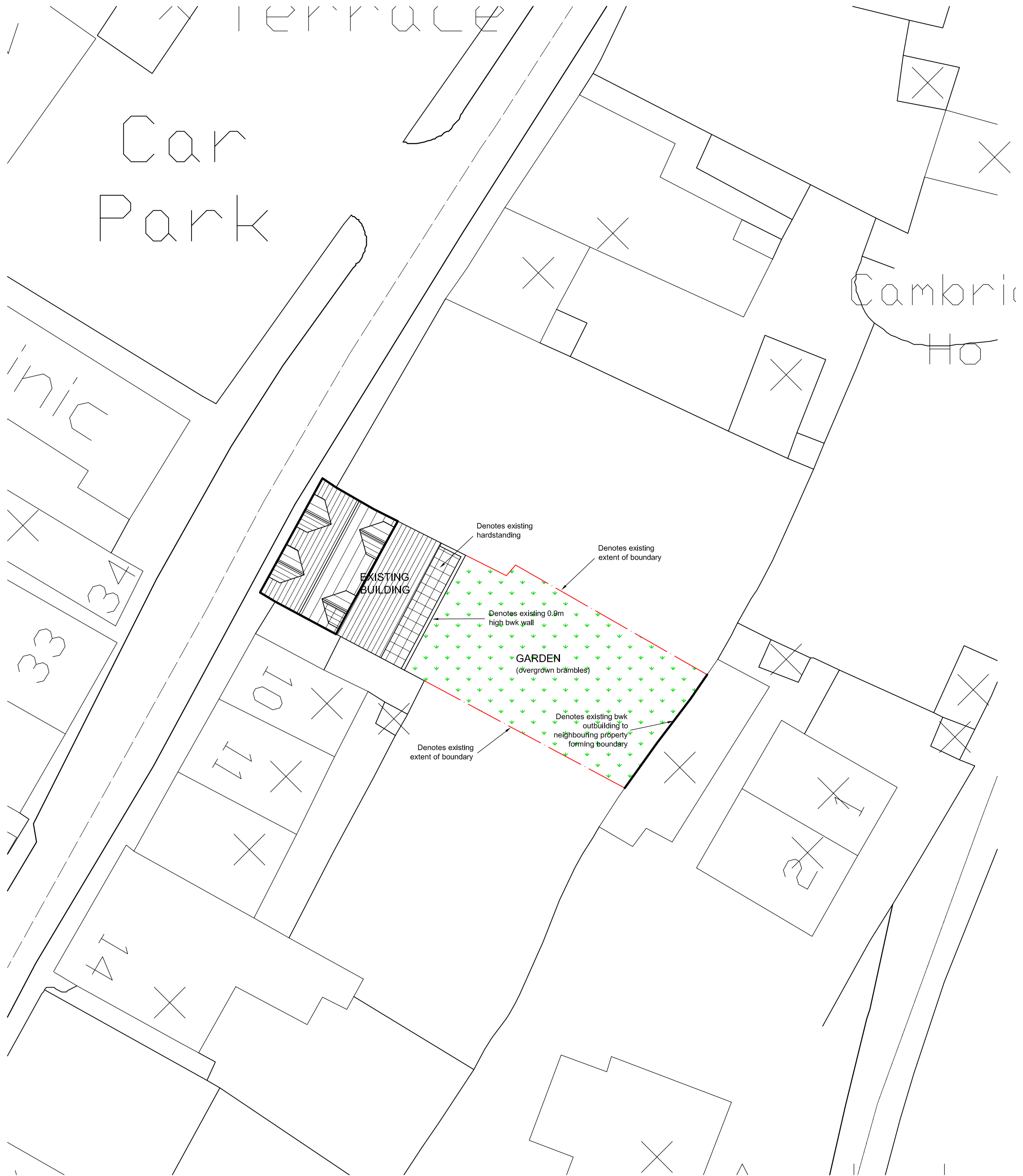
SITE PLAN (1:200)
