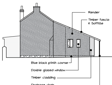
02. End Elevation 1:100 @ A1 / 1:200 @ A3
