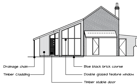
02. End Elevation 1:100 @ A1 / 1:200 @ A3
