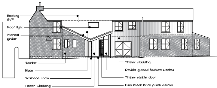
01. Front Elevation 1:100 @ A1 / 1:200 @ A3
