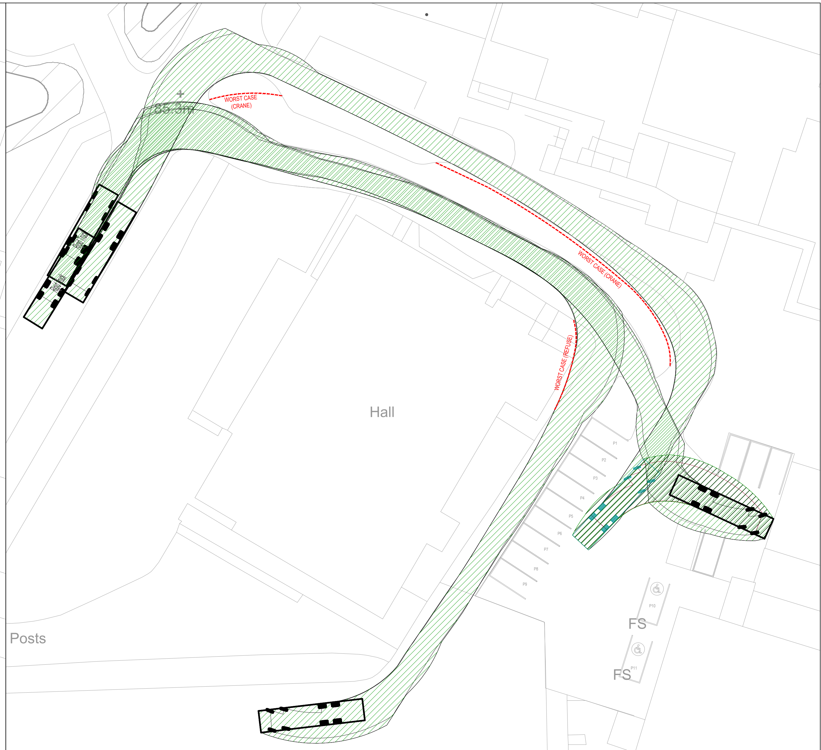
RIGID HGV
