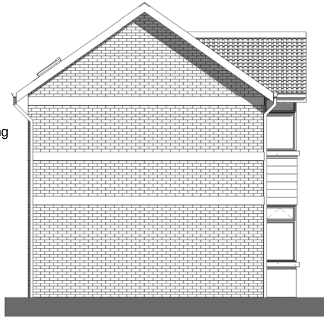
3 East 1 : 100
