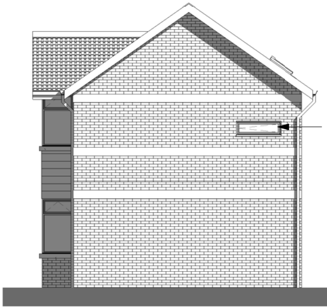
4 West 1 : 100
