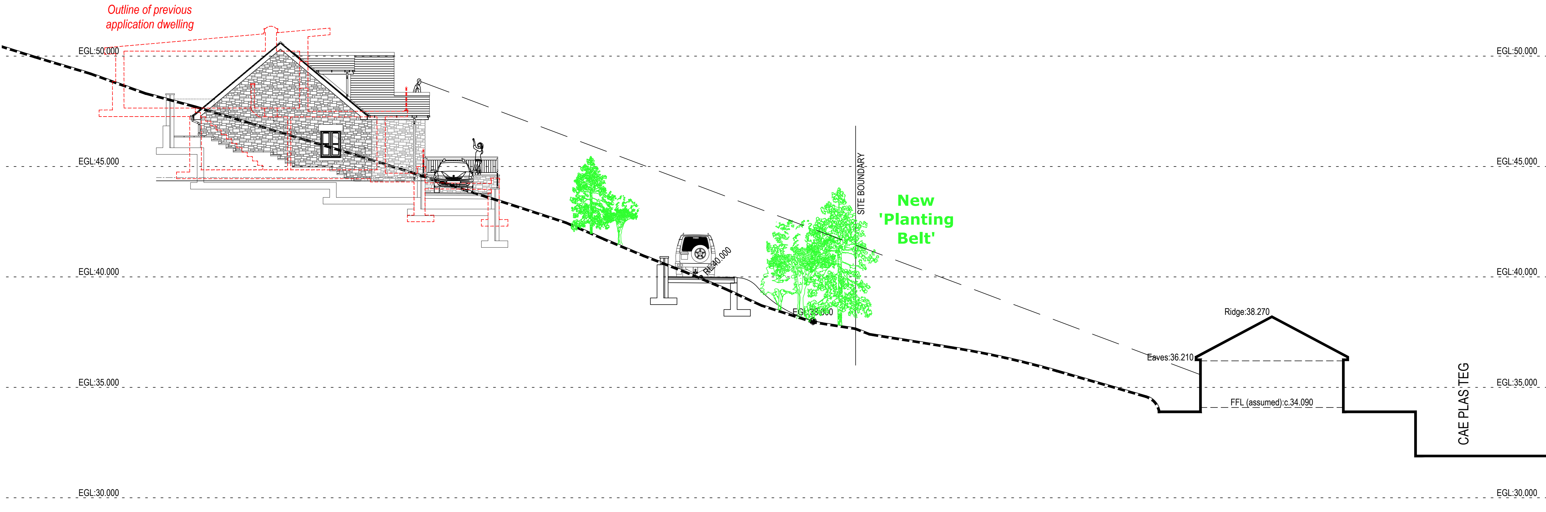
SITE CROSS SECTION A-A:
