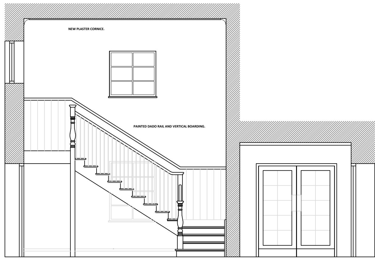
ELEVATION H. STAIRCASE (TRADE AREA 8).
