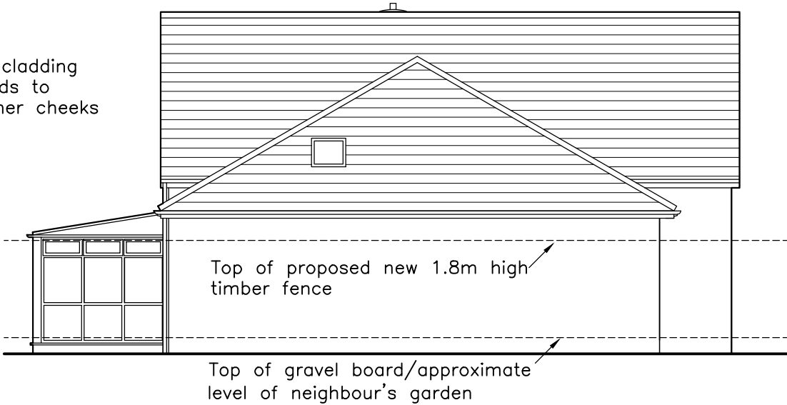
ELEVATION 2
