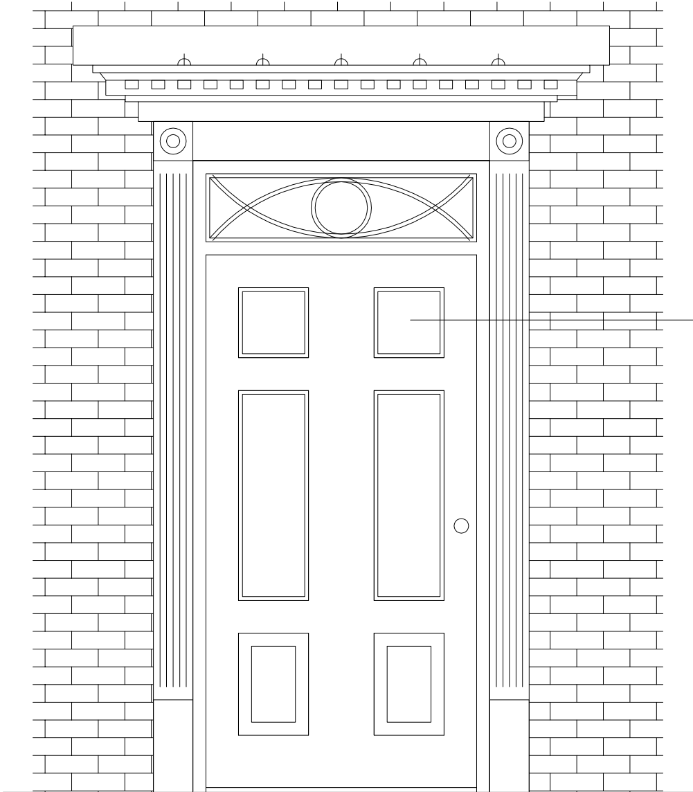
DOOR DETAIL @ 1:5
