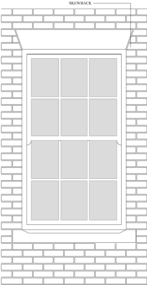
ELEVATION
