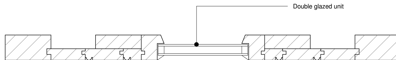
Section B - B Scale 1 : 5
