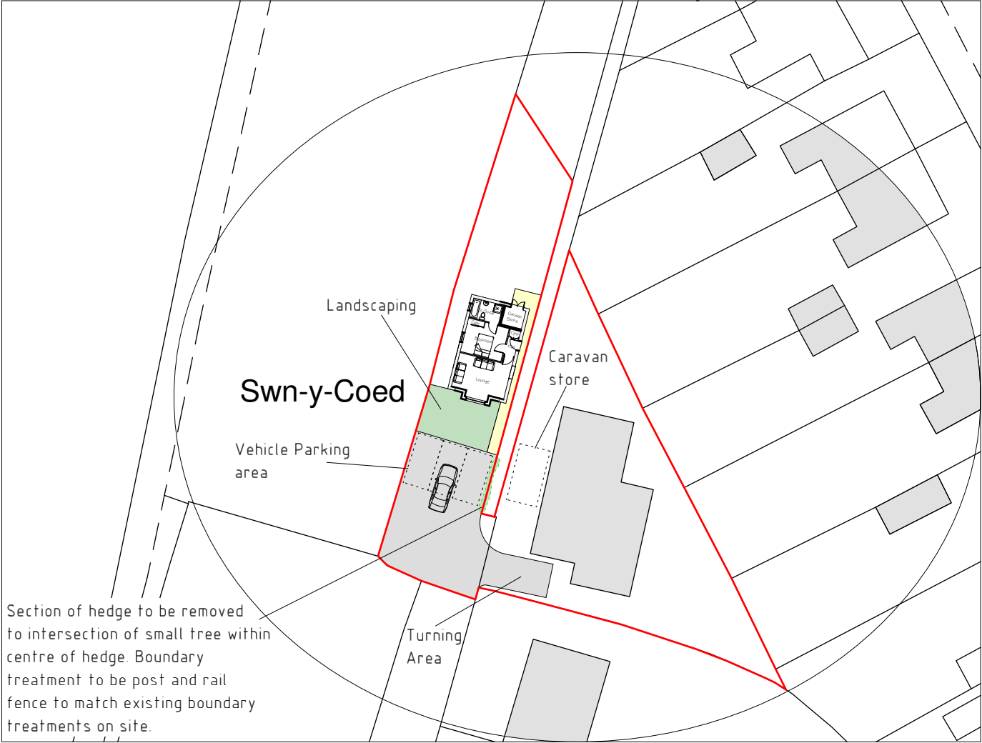
Site Plan 1:500
