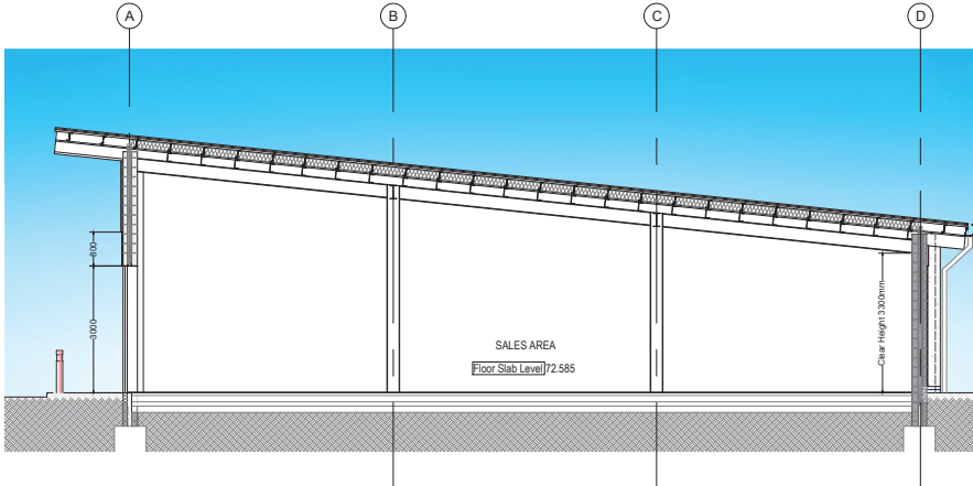
SECTION A-A 1:50
