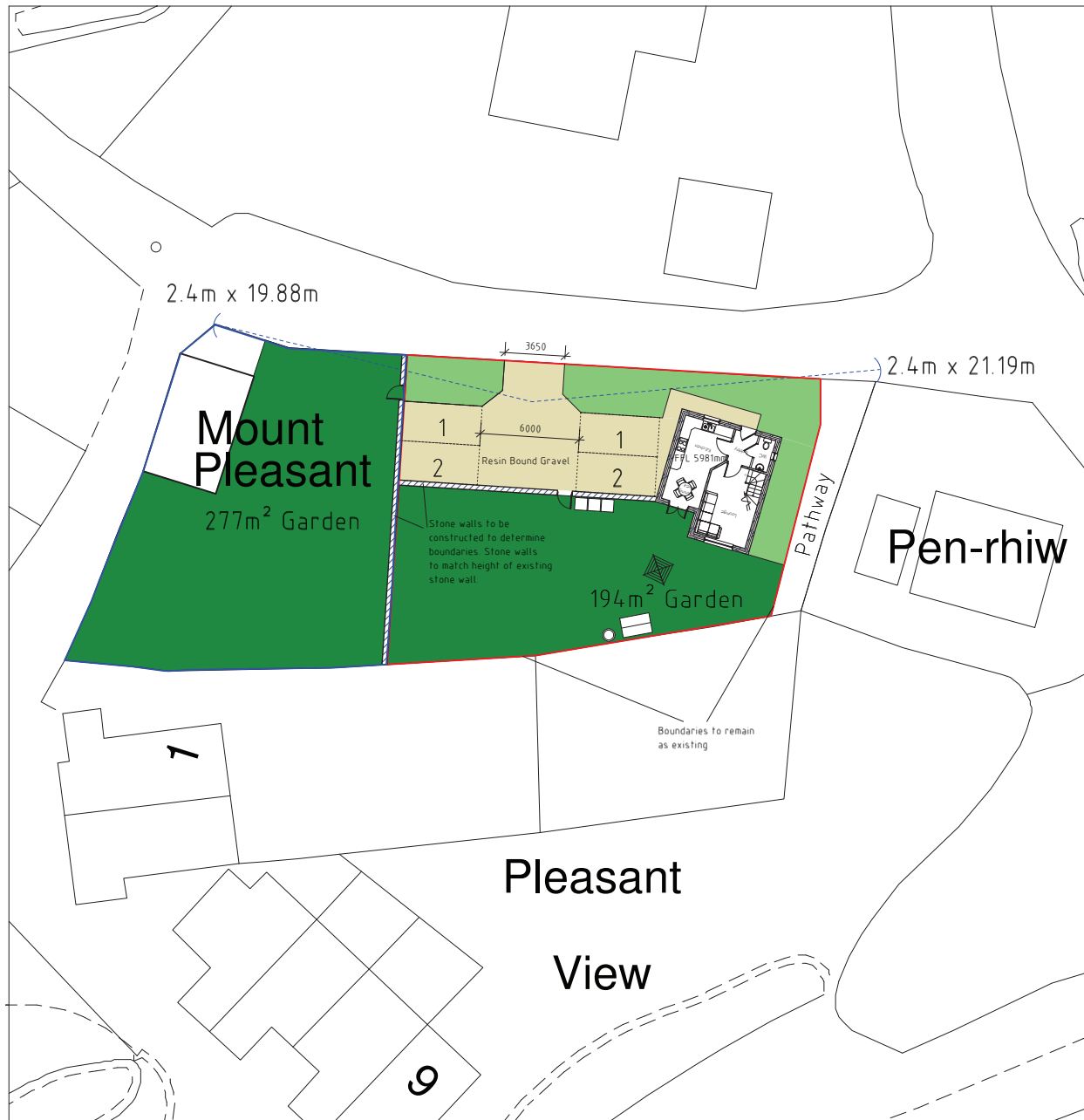
Site Plan I : 200
