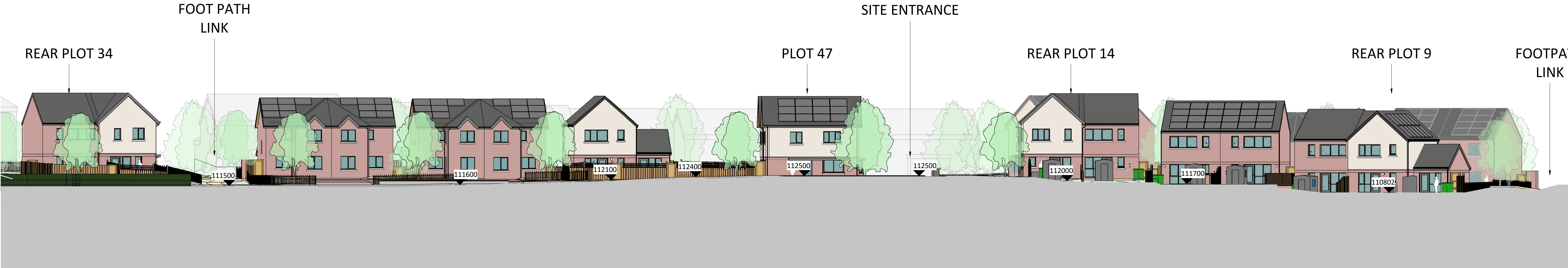
SITE SECTION A-A
