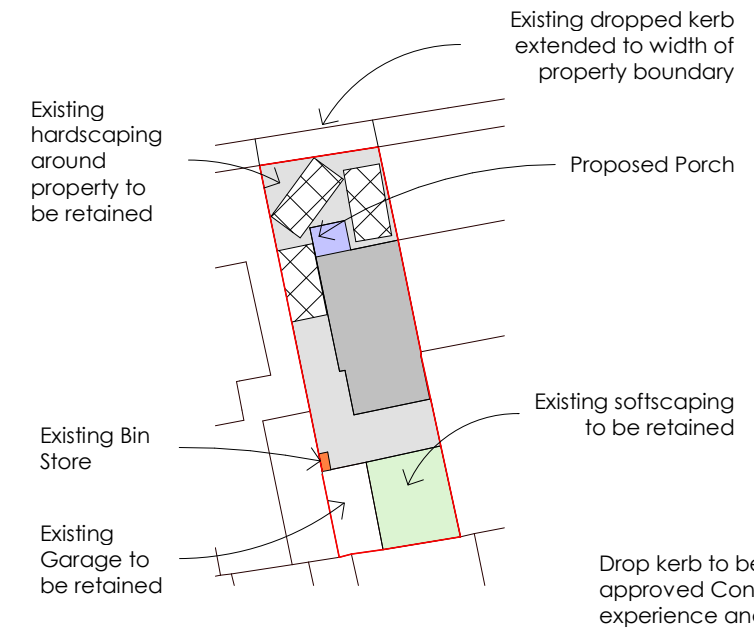
Site Plan 1 : 500
