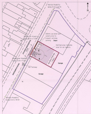
Site Plan 1:500
